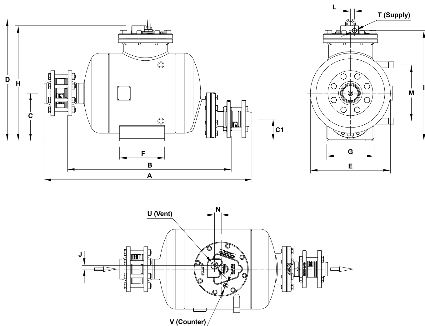
DIMENSIONS (mm) – PN 16
