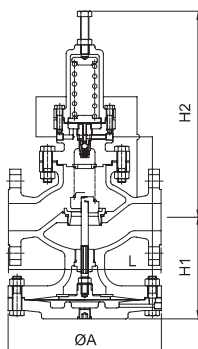
15-40A Type
