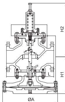
50-150A Type
